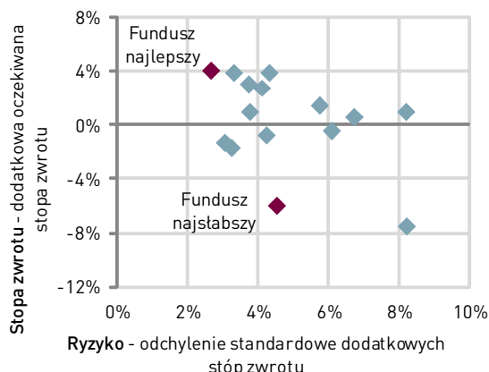
Mapa zysk/ryzyko
